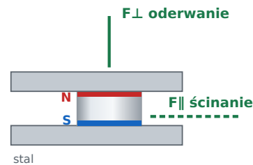
Uchwyt dwustronny dwa magnesy, obudowa dzielona F⊥ oderwanie: 4,04 kg F∥ ścinanie: 1,21 kg
