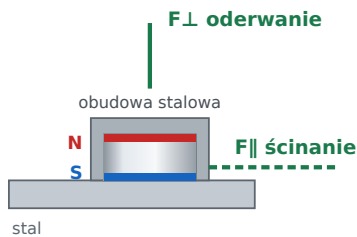
Uchwyt jednostronny magnes w obudowie stalowej F⊥ oderwanie: 0,85 kg F∥ ścinanie: 0,26 kg
