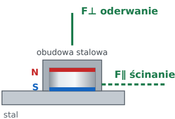
Uchwyt jednostronny magnes w obudowie stalowej F⊥ oderwanie: 131,21 kg F∥ ścinanie: 39,36 kg
