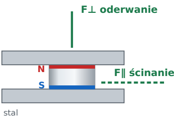
Uchwyt dwustronny dwa magnesy, obudowa dzielona F⊥ oderwanie: 124,45 kg F∥ ścinanie: 37,33 kg
