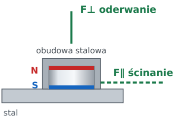
Uchwyt jednostronny magnes w obudowie stalowej F⊥ oderwanie: 138,27 kg F∥ ścinanie: 41,48 kg
