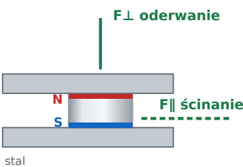
Uchwyt dwustronny dwa magnesy, obudowa dzielona F⊥ oderwanie: 71,53 kg F∥ ścinanie: 21,46 kg
