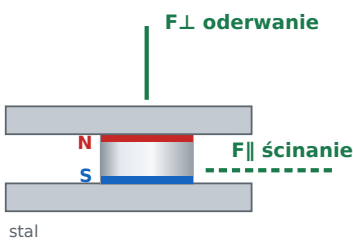
Uchwyt dwustronny dwa magnesy, obudowa dzielona F⊥ oderwanie: 44,76 kg F∥ ścinanie: 13,43 kg
