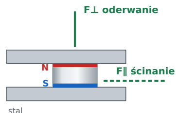
Uchwyt dwustronny dwa magnesy, obudowa dzielona F⊥ oderwanie: 6,62 kg F∥ ścinanie: 1,99 kg
