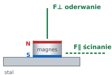
Magnes goły magnes bez obudowy F⊥ oderwanie: 3,39 kg F∥ ścinanie: 1,02 kg
