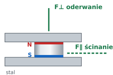
Uchwyt dwustronny dwa magnesy, obudowa dzielona F⊥ oderwanie: 3,28 kg F∥ ścinanie: 0,98 kg
