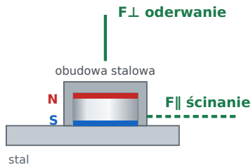
Uchwyt jednostronny magnes w obudowie stalowej F⊥ oderwanie: 2,14 kg F∥ ścinanie: 0,64 kg
