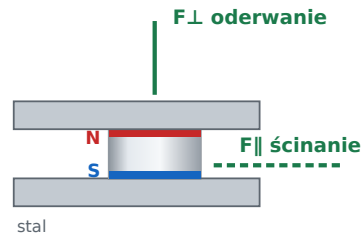
Uchwyt dwustronny dwa magnesy, obudowa dzielona F⊥ oderwanie: 1,93 kg F∥ ścinanie: 0,58 kg
