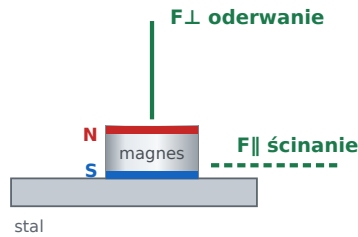
Magnes goły magnes bez obudowy F⊥ oderwanie: 0,82 kg F∥ ścinanie: 0,25 kg
