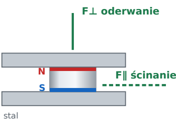
Uchwyt dwustronny dwa magnesy, obudowa dzielona F⊥ oderwanie: 77,81 kg F∥ ścinanie: 23,34 kg
