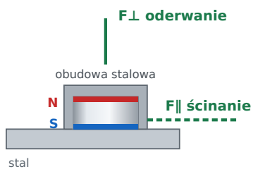
Uchwyt jednostronny magnes w obudowie stalowej F⊥ oderwanie: 69,63 kg F∥ ścinanie: 20,89 kg
