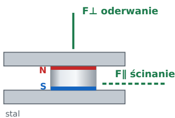
Uchwyt dwustronny dwa magnesy, obudowa dzielona F⊥ oderwanie: 26,70 kg F∥ ścinanie: 8,01 kg
