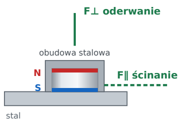
Uchwyt jednostronny magnes w obudowie stalowej F⊥ oderwanie: 5,69 kg F∥ ścinanie: 1,71 kg
