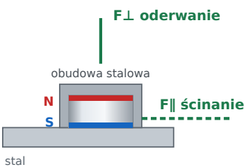
Uchwyt jednostronny magnes w obudowie stalowej F⊥ oderwanie: 37,67 kg F∥ ścinanie: 11,30 kg
