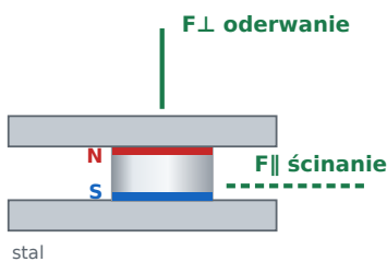
Uchwyt dwustronny dwa magnesy, obudowa dzielona F⊥ oderwanie: 33,90 kg F∥ ścinanie: 10,17 kg
