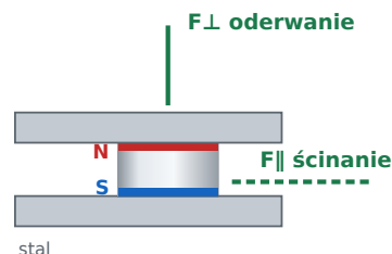
Uchwyt dwustronny dwa magnesy, obudowa dzielona F⊥ oderwanie: 3,98 kg F∥ ścinanie: 1,19 kg
