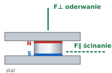
Uchwyt dwustronny dwa magnesy, obudowa dzielona F⊥ oderwanie: 13,16 kg F∥ ścinanie: 3,95 kg
