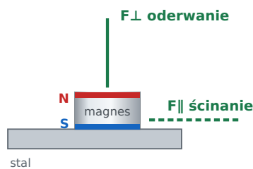
Magnes goły magnes bez obudowy F⊥ oderwanie: 9,42 kg F∥ ścinanie: 2,82 kg
