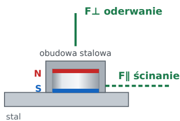
Uchwyt jednostronny magnes w obudowie stalowej F⊥ oderwanie: 19,20 kg F∥ ścinanie: 5,76 kg
