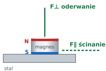
Magnes goły magnes bez obudowy F⊥ oderwanie: 7,25 kg F∥ ścinanie: 2,17 kg
