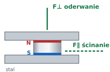
Uchwyt dwustronny dwa magnesy, obudowa dzielona F⊥ oderwanie: 17,28 kg F∥ ścinanie: 5,19 kg
