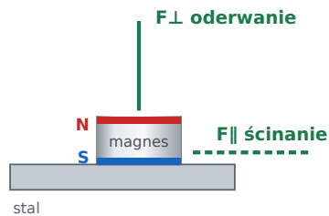
Magnes goły magnes bez obudowy F⊥ oderwanie: 9,48 kg F∥ ścinanie: 2,84 kg
