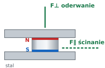
Uchwyt dwustronny dwa magnesy, obudowa dzielona F⊥ oderwanie: 22,61 kg F∥ ścinanie: 6,78 kg
