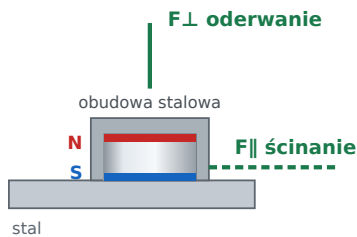
Uchwyt jednostronny magnes w obudowie stalowej F⊥ oderwanie: 7,52 kg F∥ ścinanie: 2,26 kg
