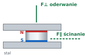
Uchwyt dwustronny dwa magnesy, obudowa dzielona F⊥ oderwanie: 6,77 kg F∥ ścinanie: 2,03 kg
