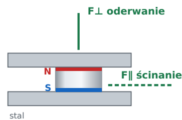
Uchwyt dwustronny dwa magnesy, obudowa dzielona F⊥ oderwanie: 15,88 kg F∥ ścinanie: 4,76 kg
