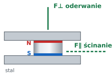
Uchwyt dwustronny dwa magnesy, obudowa dzielona F⊥ oderwanie: 4,76 kg F∥ ścinanie: 1,43 kg
